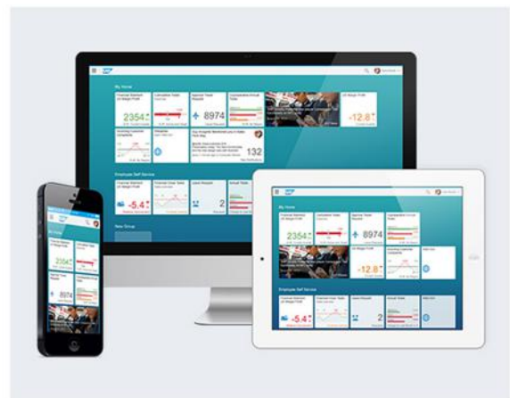
SAP FIORI
